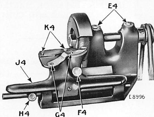
Fig. 22. Knife Grinder 234746
